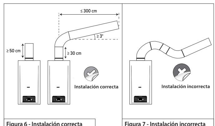
Figura 6 - Instalación correcta
