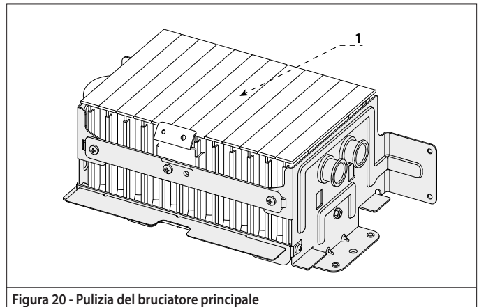
Figura 20 - Pulizia del bruciatore principale
