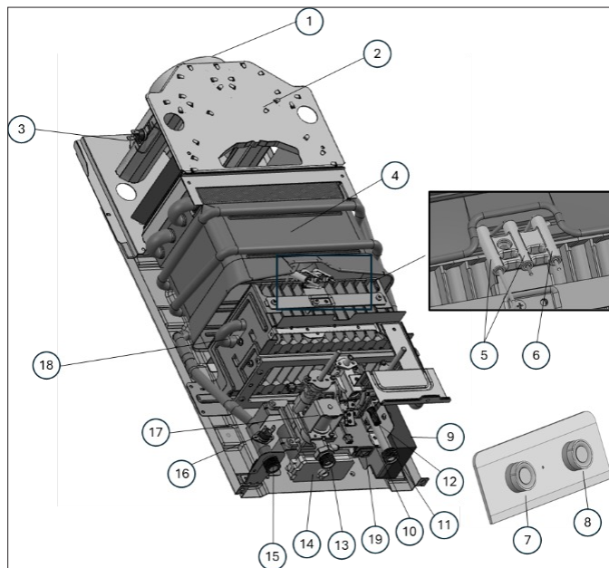
Figura 3 - Vista complessiva
