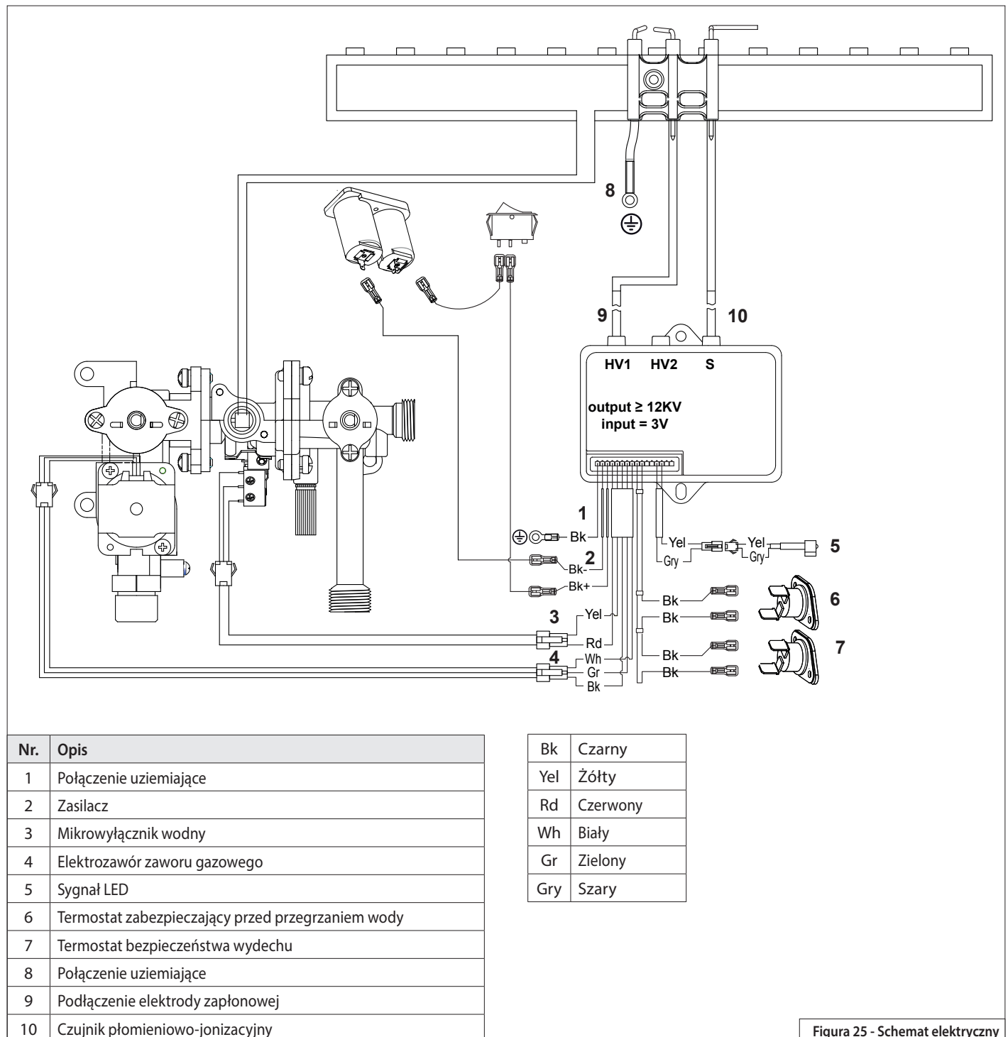
Figura 25 - Schemat elektryczny
