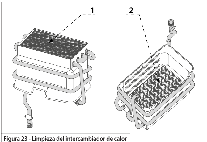
Figura 23 - Limpieza del intercambiador de calor
