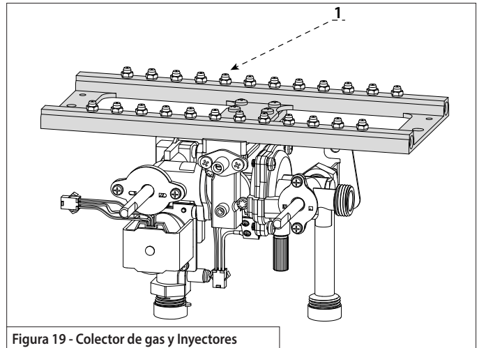
Figura 19 - Colector de gas y Inyectores
