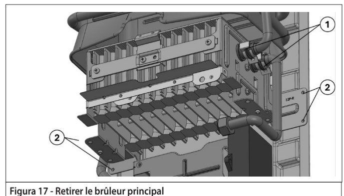
Figura 17 - Retirer le brûleur principal
