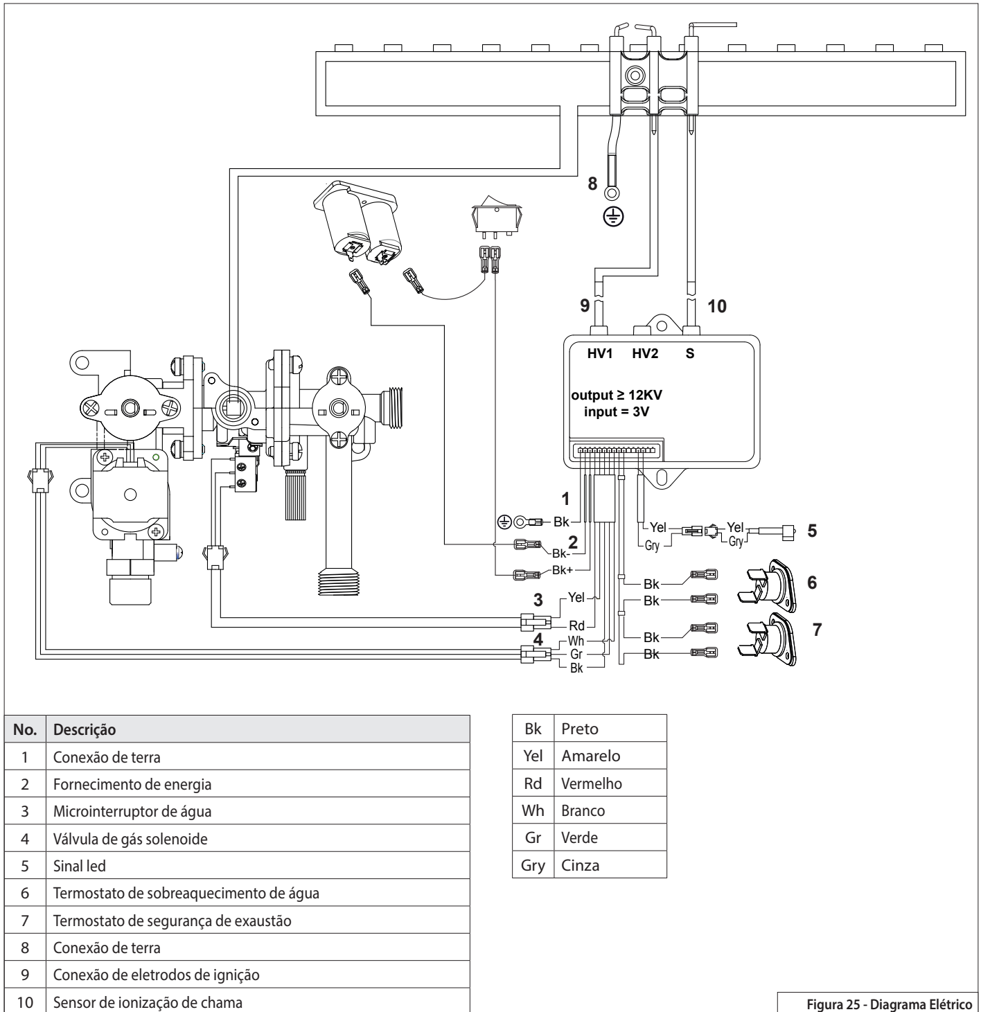
Figura 25 - Diagrama Elétrico
