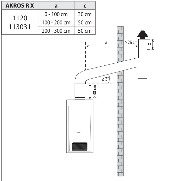
Figura 8 - Configuraciones de instalación de los tubos de evacuación
