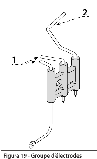
Figura 19 - Groupe d'électrodes
