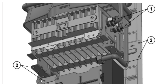
Figura 19 - Zdejmij główny palnik
