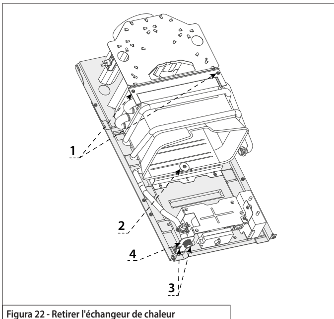
Figura 22 - Retirer l'échangeur de chaleur
