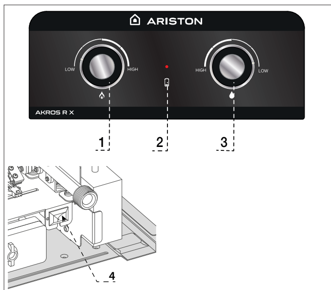
Figura 1 - Panneau de commande et bouton marche/arrêt
