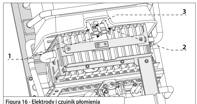
Figura 16 - Elektrody i czujnik płomienia
