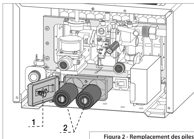
Figura 2 - Remplacement des piles
