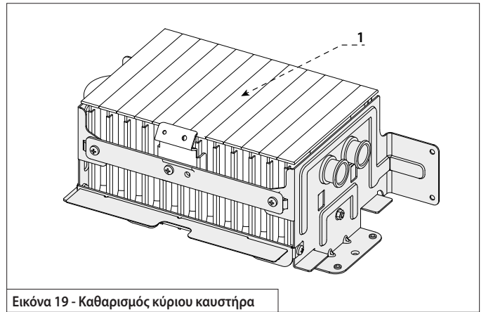
Εικόνα 19 - Καθαρισμός κύριου καυστήρα
