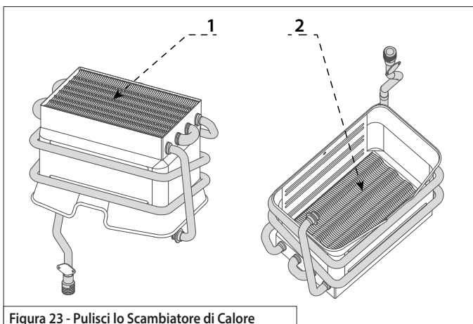
Figura 23 - Pulisci lo Scambiatore di Calore
