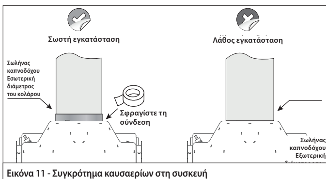
Εικόνα 11 - Συγκρότημα καυσαερίων στη συσκευή
