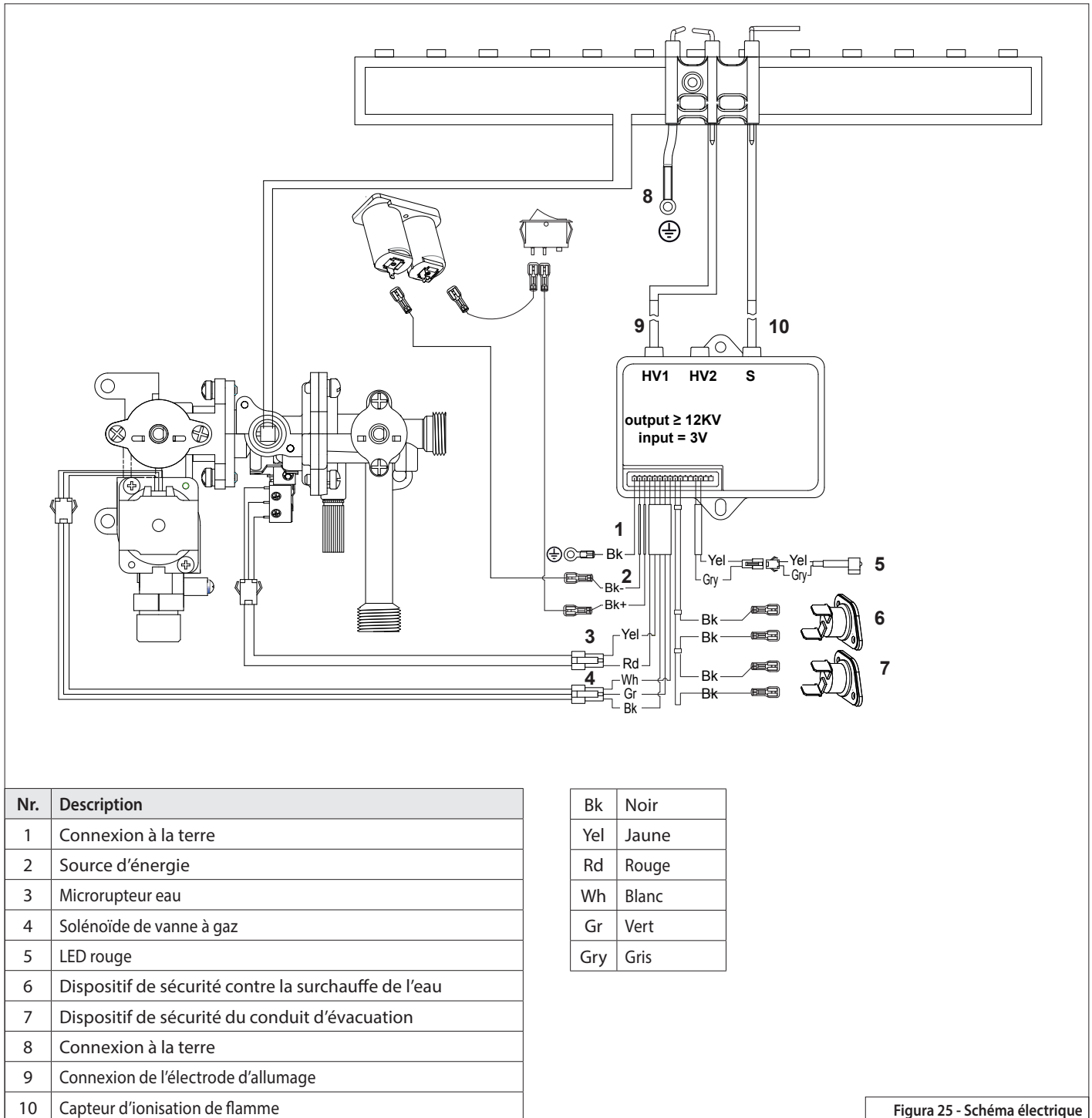
Figura 25 - Schéma électrique
