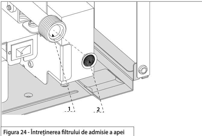
Figura 24 - Întreținerea filtrului de admisie a apei
