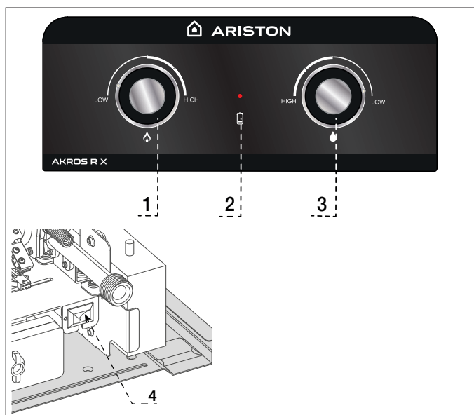
Figura 1 - Panel sterowania i przycisk włączania/wyłączania
