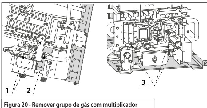
Figura 20 - Remover grupo de gás com multiplicador
