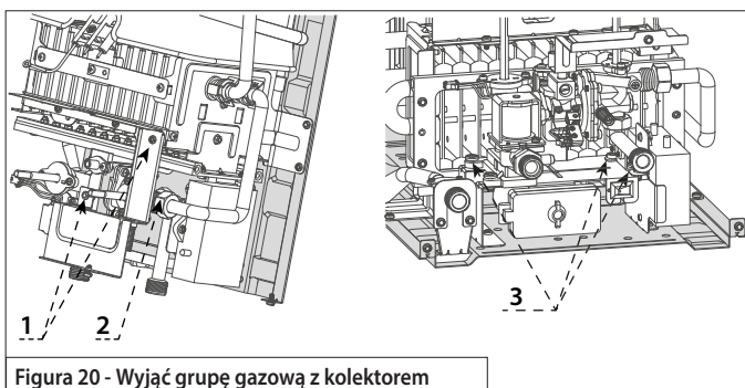
Figura 20 - Wyjąć grupę gazową z kolektorem
