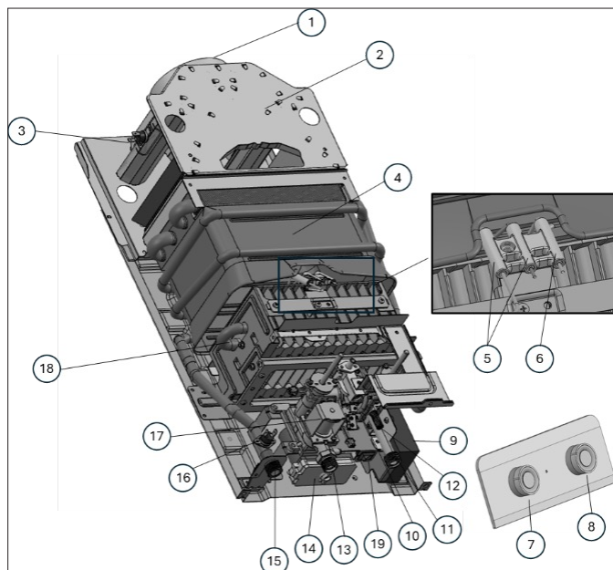
Figura 3 - Vue globale
