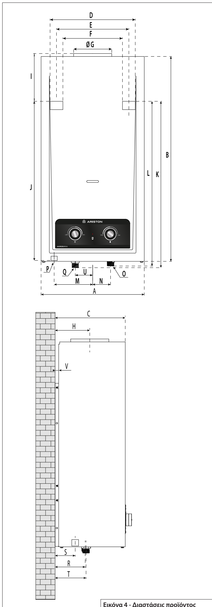
Εικόνα 4 - Διαστάσεις προϊόντος
