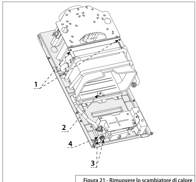
Figura 21 - Rimuovere lo scambiatore di calore
