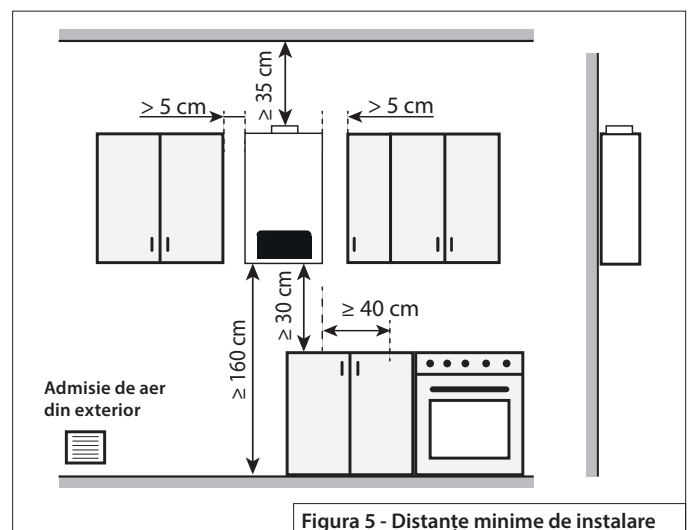
Figura 5 - Distanțe minime de instalare
