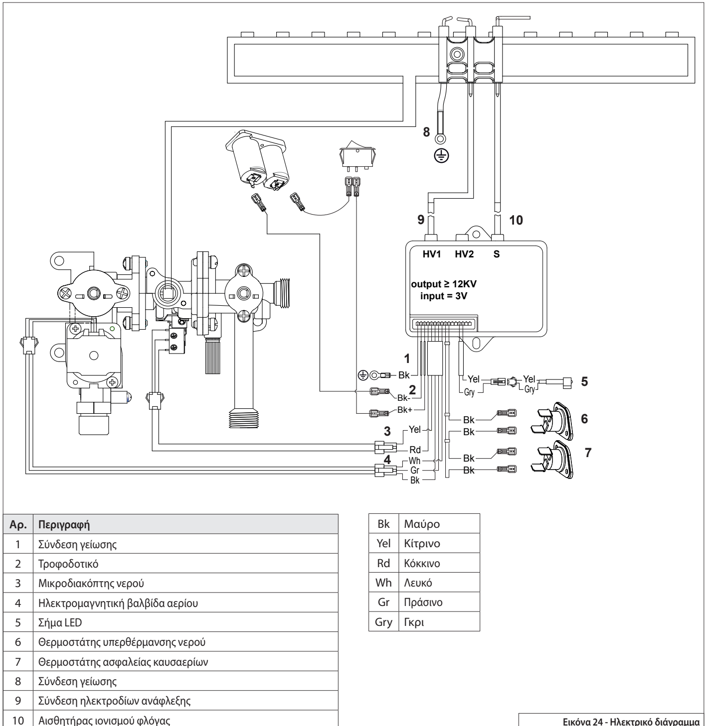
Εικόνα 24 - Ηλεκτρικό διάγραμμα
