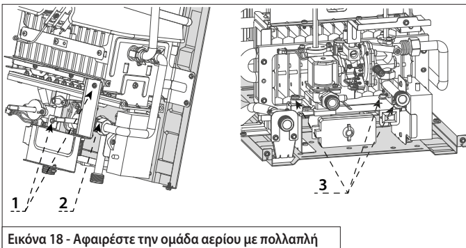
Εικόνα 18 - Αφαιρέστε την ομάδα αερίου με πολλαπλή
