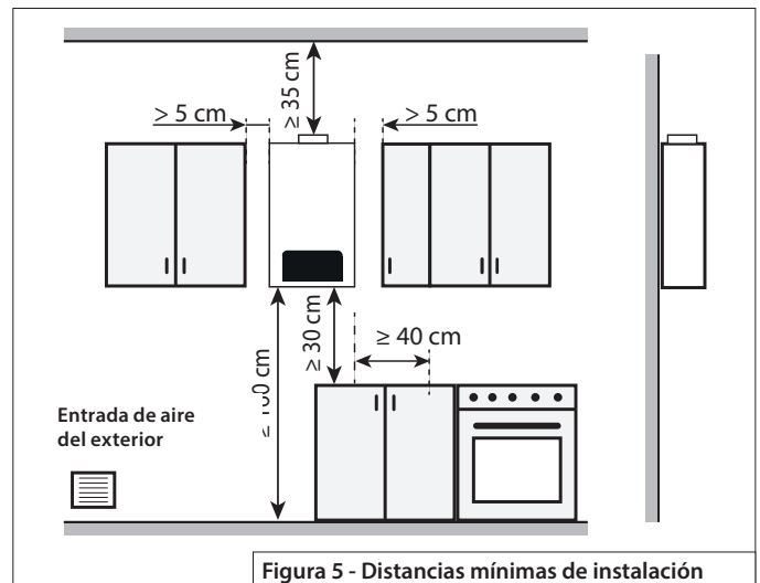
Figura 5 - Distancias mínimas de instalación
