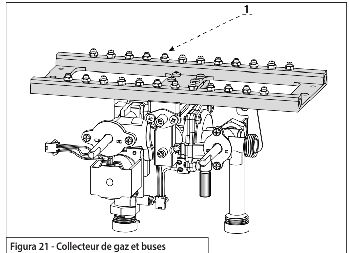
Figura 21 - Collecteur de gaz et buses
