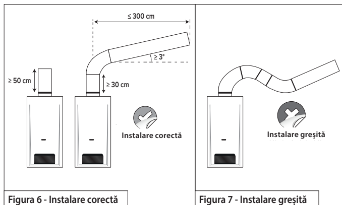
Figura 6 - Instalare corectă
