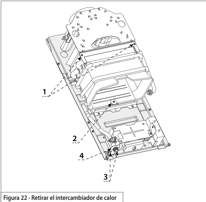
Figura 22 - Retirar el intercambiador de calor
