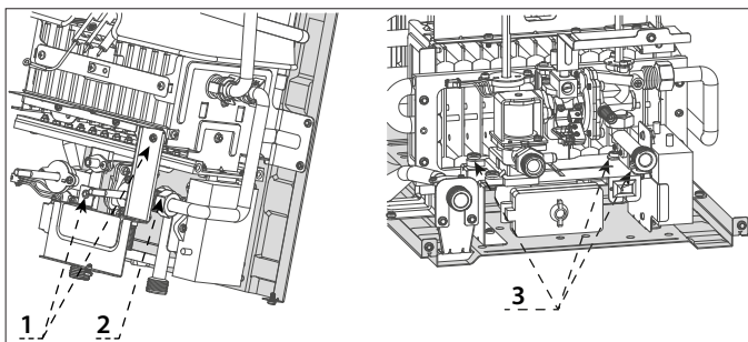
Figura 22 - Îndepărtați grupul de gaz cu colectorul
