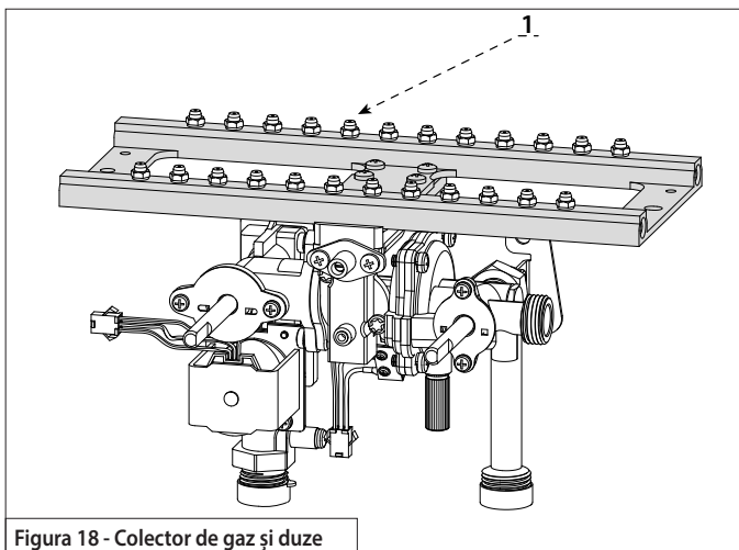
Figura 18 - Colector de gaz și duze
