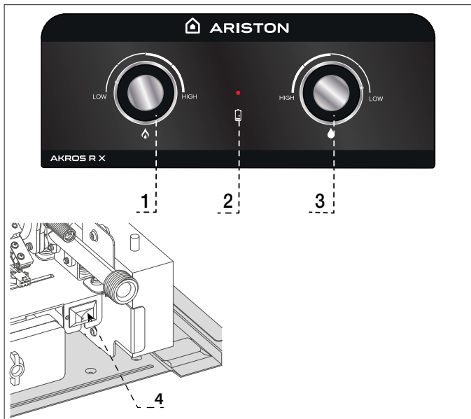
Εικόνα 1 - Πίνακας ελέγχου και κουμπί ενεργοποίησης/απενεργοποίησης
