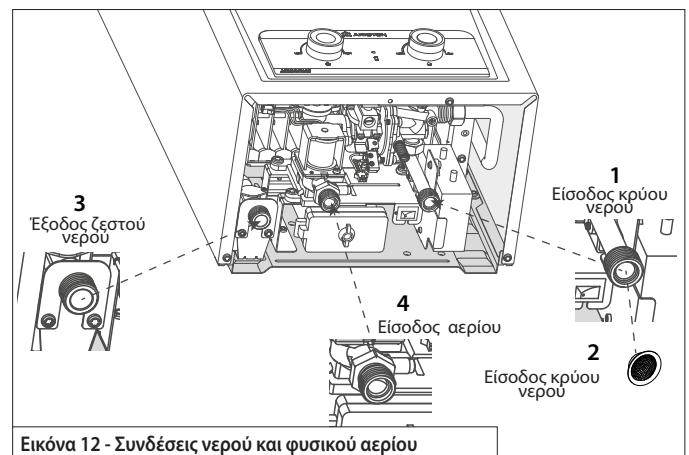
Εικόνα 12 - Συνδέσεις νερού και φυσικού αερίου
