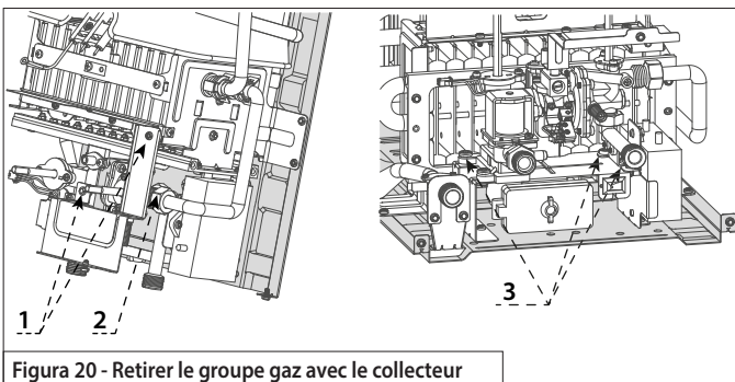
Figura 20 - Retirer le groupe gaz avec le collecteur
