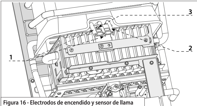
Figura 16 - Electrodo de encendido y sensor de llama
