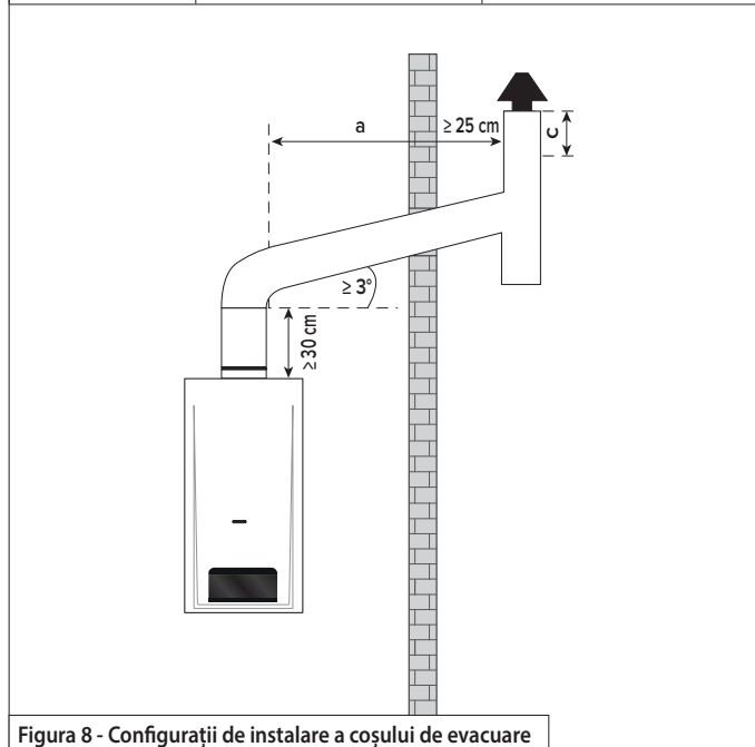
Figura 8 - Configurații de instalare a coșului de evacuare
