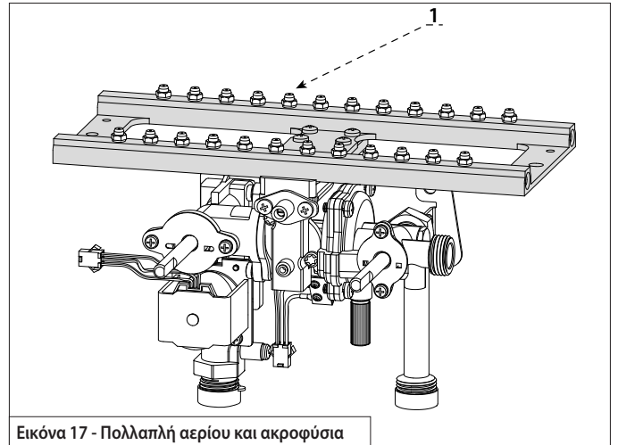
Εικόνα 17 - Πολλαπλή αερίου και ακροφύσια
