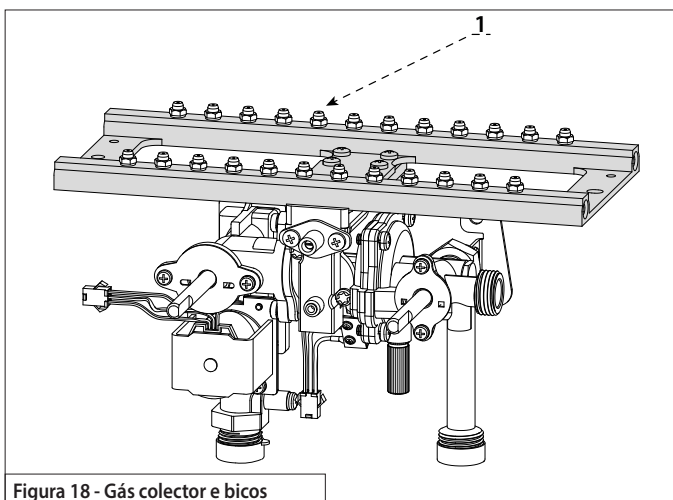
Figura 18 - Gás colector e bicos
