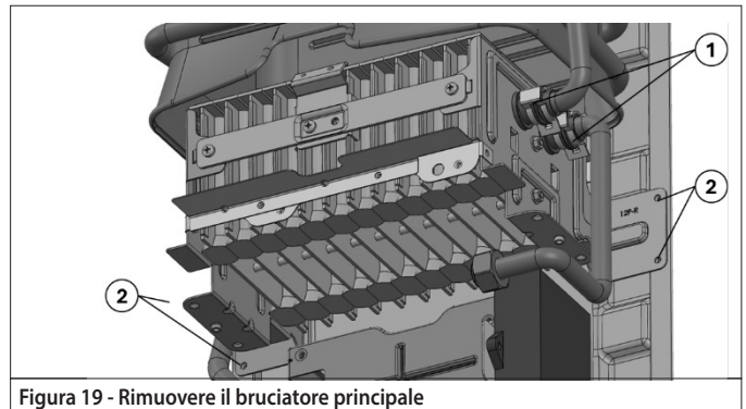
Figura 19 - Rimuovere il bruciatore principale
