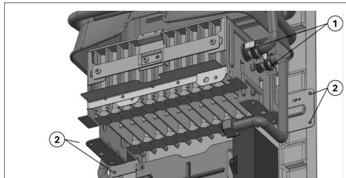
Figura 19 - Scoateți arzătorul principal
