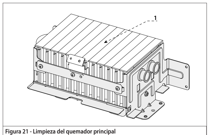
Figura 21 - Limpieza del quemador principal
