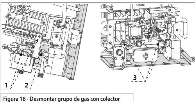
Figura 18 - Desmontar grupo de gas con colector
