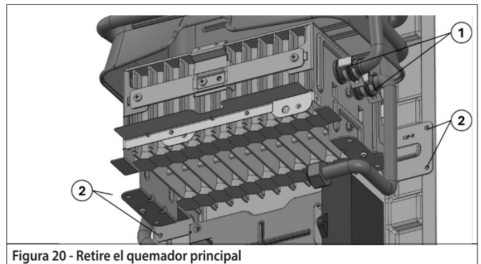
Figura 20 - Retire el quemador principal
