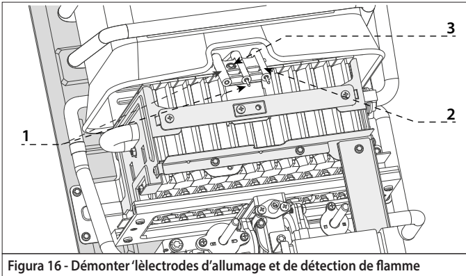
Figura 16 - Démontez les électrodes d'allumage et de détection de flamme
