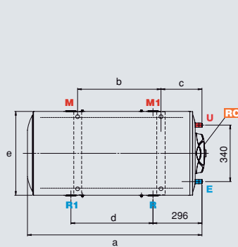
Instalação horizontal
