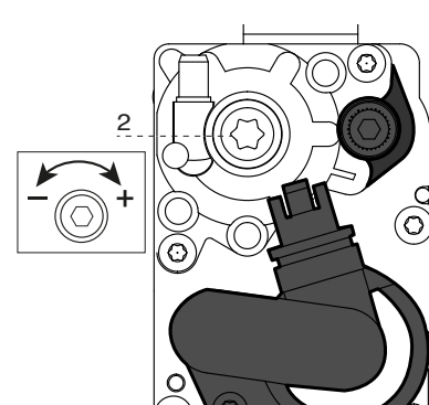
Válvula de gas 8205 / Válvula de gás 8205
